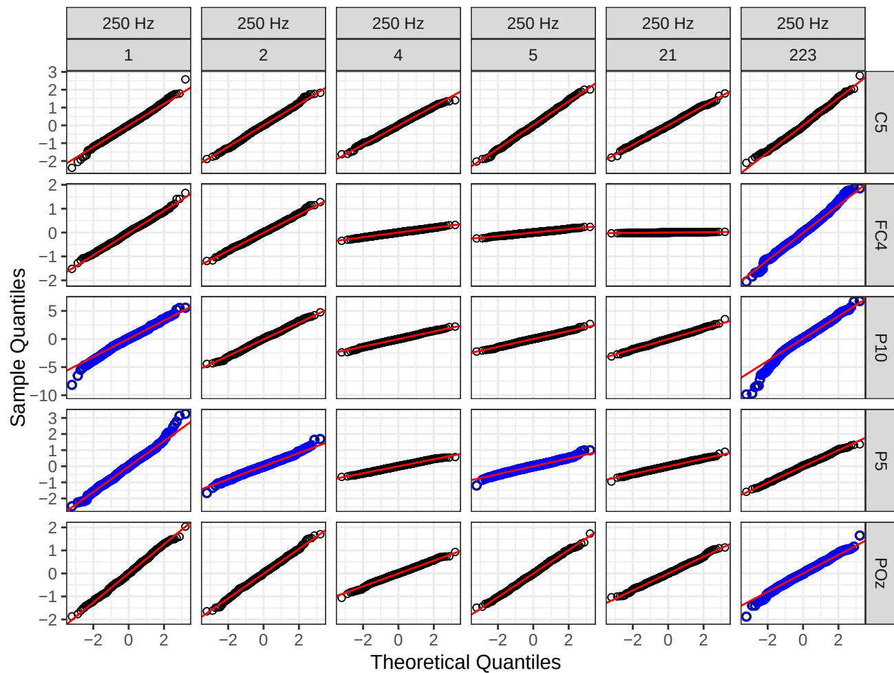
Q-Q plot p=1
